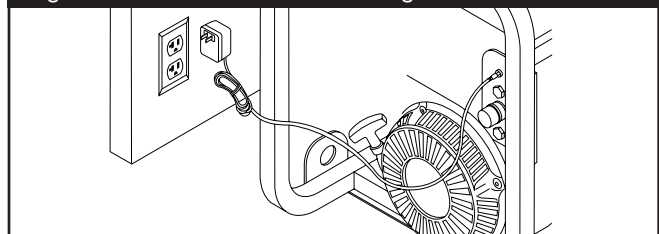
Figura 17 — Enchufe Hembra del Cargador de Flotación
